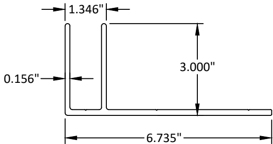
JAMB F-ANCHOR (WINDOW WALL) E1-7025
