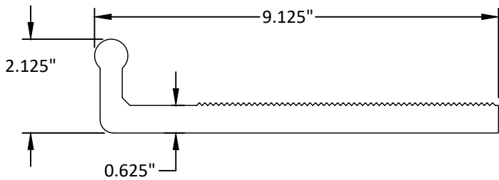
L-ANCHOR E1-3907
