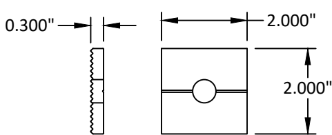
LOCK WASHER E1-3908
