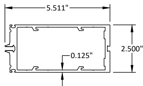
5 1/4" JAMB MULLION E9-7098
